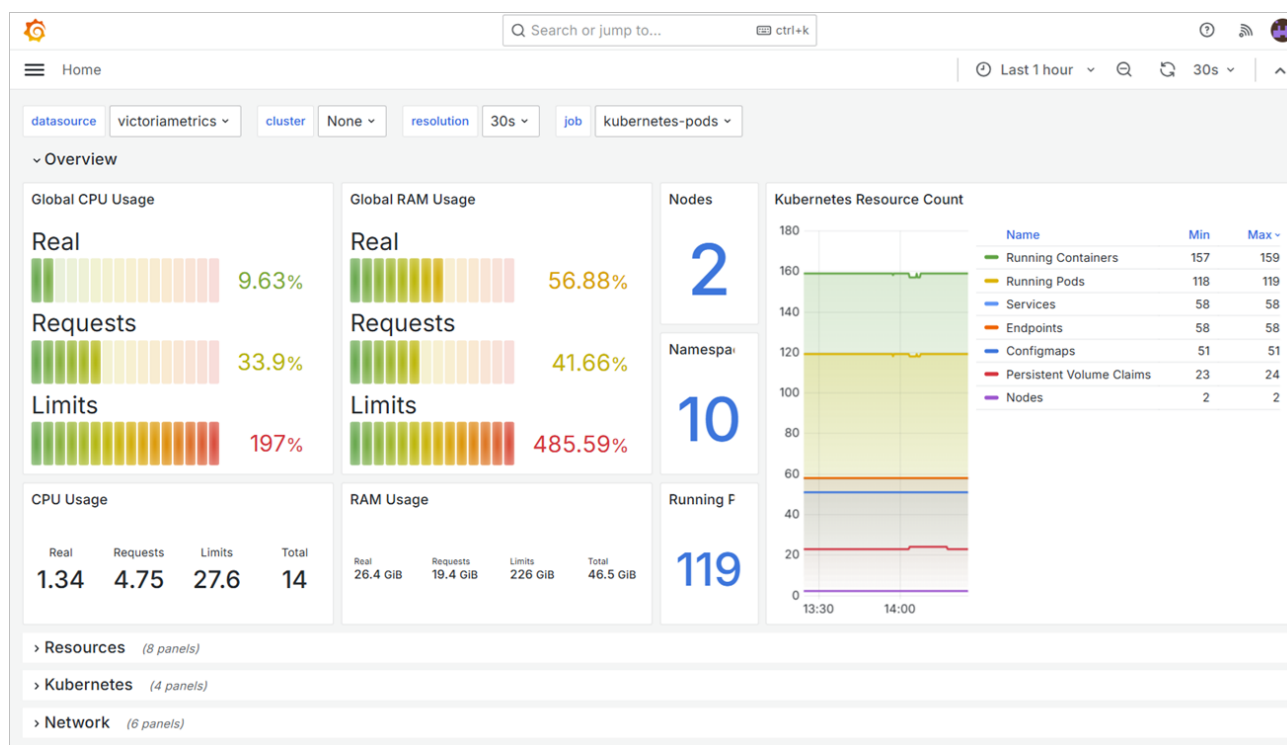
Рисунок 21. Мониторинг системных ресурсов в Grafana
