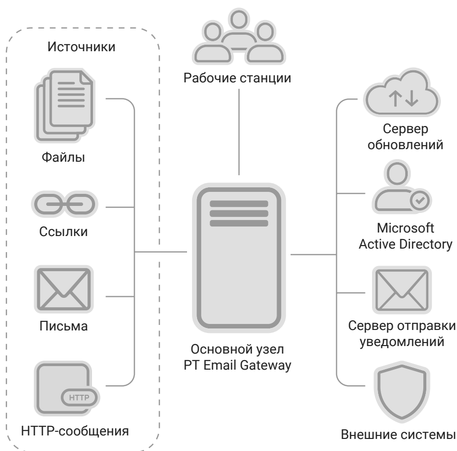
Рисунок 1. Базовая конфигурация PT Email Gateway
