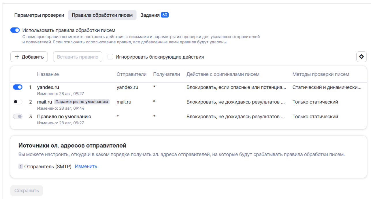
Рисунок 17. Вкладка Правила обработки писем
