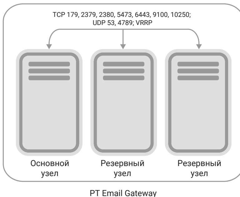
Рисунок 3. Порты взаимодействия узлов PT Email Gateway
