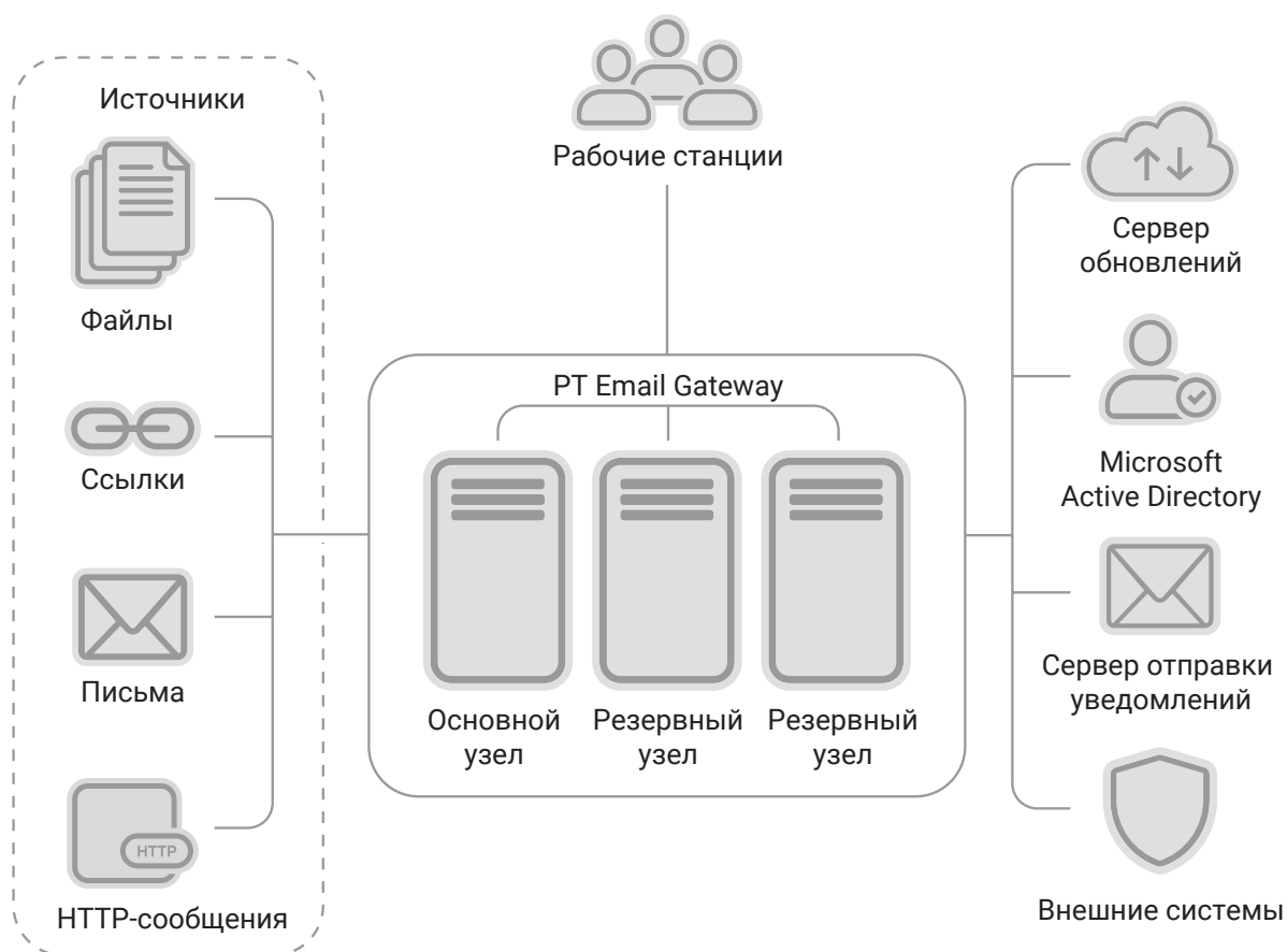
Рисунок 2. Отказоустойчивый кластер PT Email Gateway
