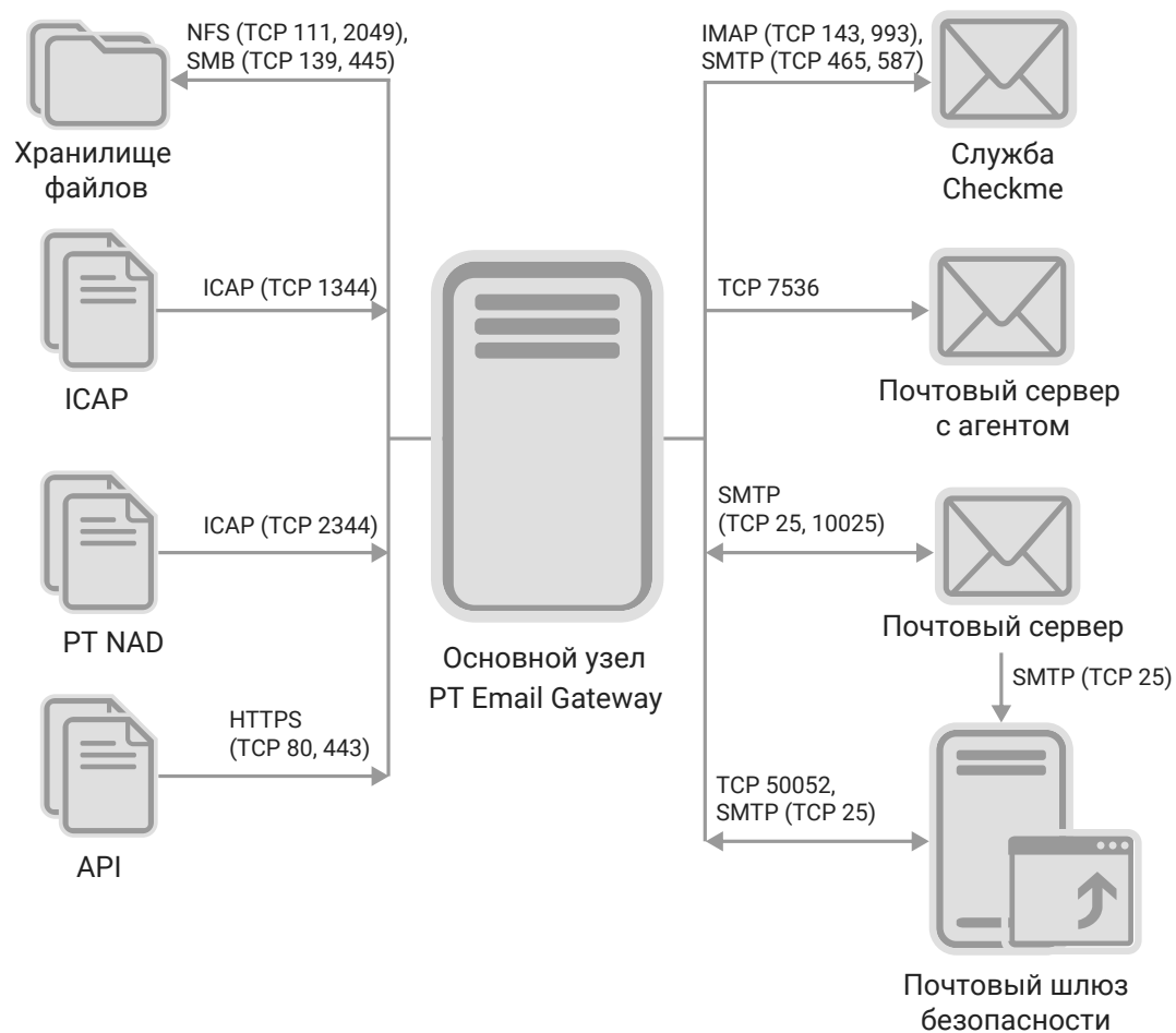
Рисунок 5. Порты взаимодействия PT Email Gateway с источниками
