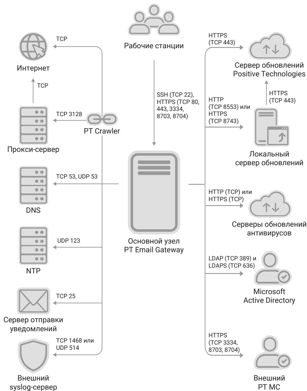
Рисунок 4. Порты взаимодействия основного узла PT Email Gateway с компонентами информационной системы
