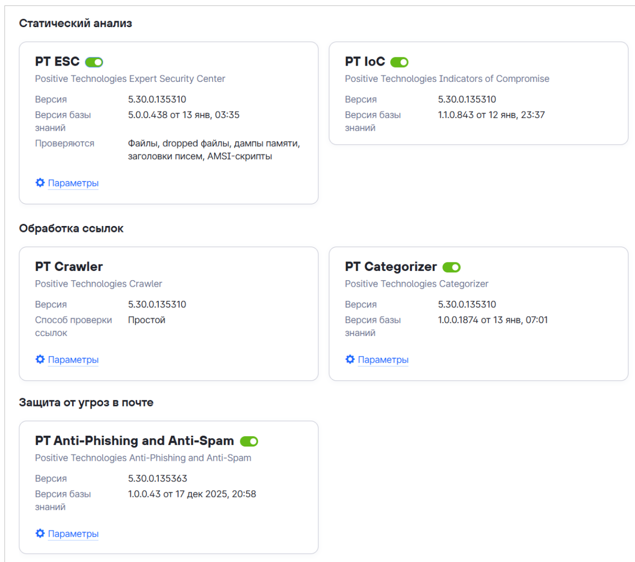
Рисунок 2. Страница Экспертиза PT
